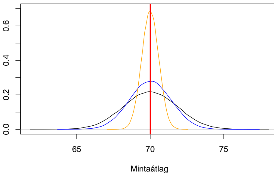
4.2. ábra. A mintavételi eloszlás függése a mintanagyságtól.
